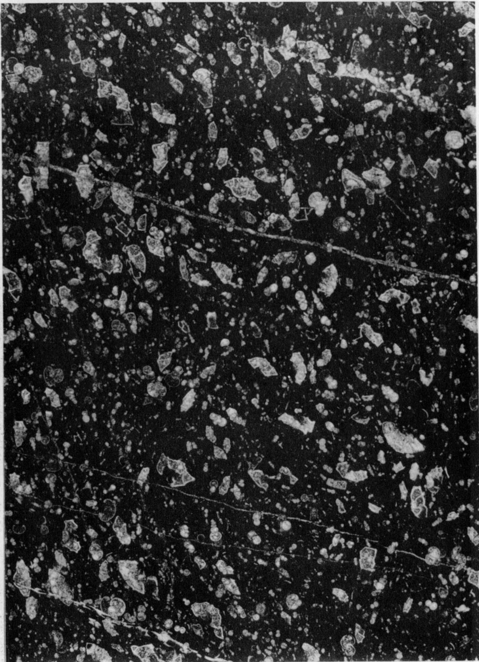
Fig. 3. Scaglia con Globotruncana linnei (D'ORB.) e Globotruncana stuarti (DE LAPP.) = Zona 1 b'.
