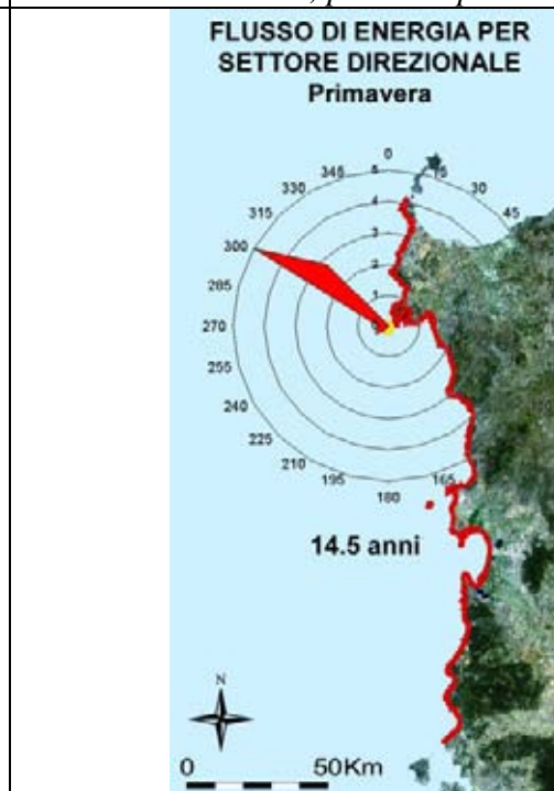
Fig 3.12.12 Media annuale del flusso lordo di energia in Kw/m per settori direzionali di 15^\circ - tratto costiero da C.po del Falcone a C.po Altano- dati triorari, periodo: primavera
