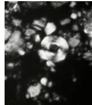
Nannofossile
