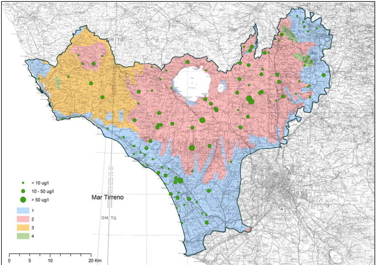
Fig. 16 - Carta delle concentrazioni dell'arsenico. Schema geolitologico: 1 = formazioni sedimentarie plio-quadernarie; 2 = vulcaniti plio-quadernarie; 3 = complesso dei flysch; 4 = formazioni carbonatiche meso-cenozoiche. - Arsenic concentration map. Geolithological sketch: 1 = Plio-Quaternary sedimentary formations; 2 = Plio-Quaternary volcanites; 3 = flysch complex; 4 = Meso-Cenozoic calcareous formations.
