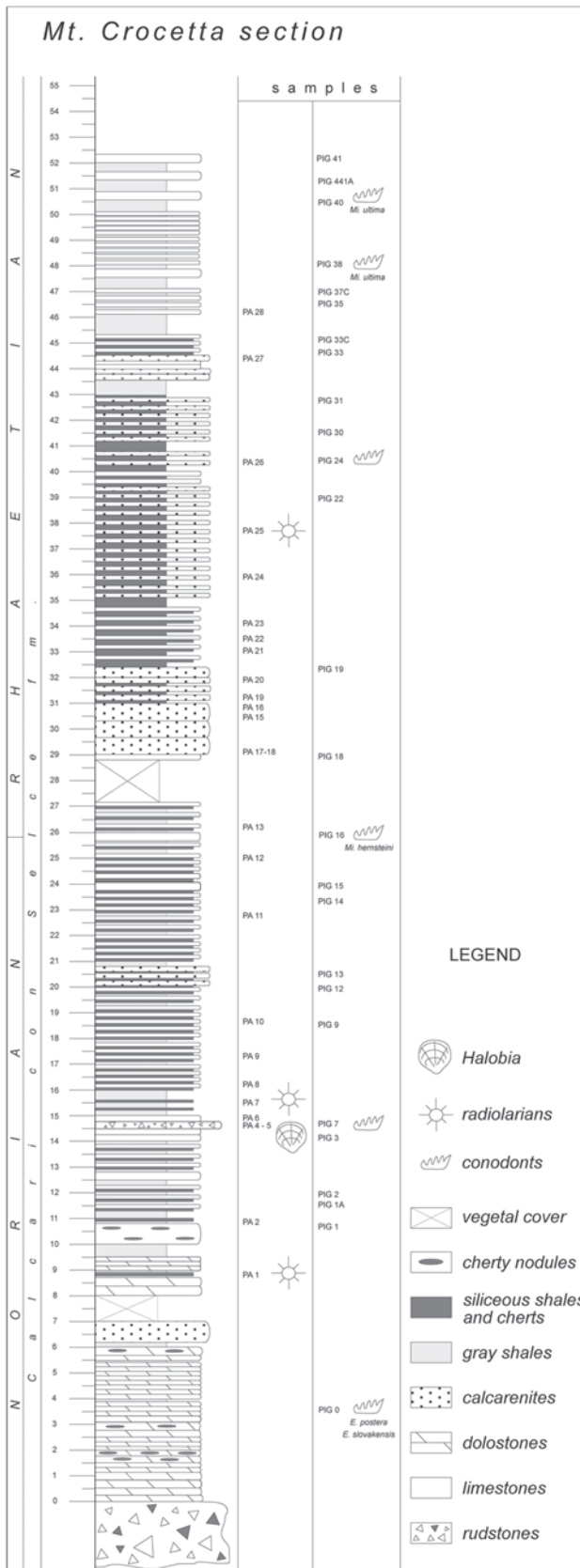
Log litostратigrafico della sezione del M. Crocetta (Pignola).
