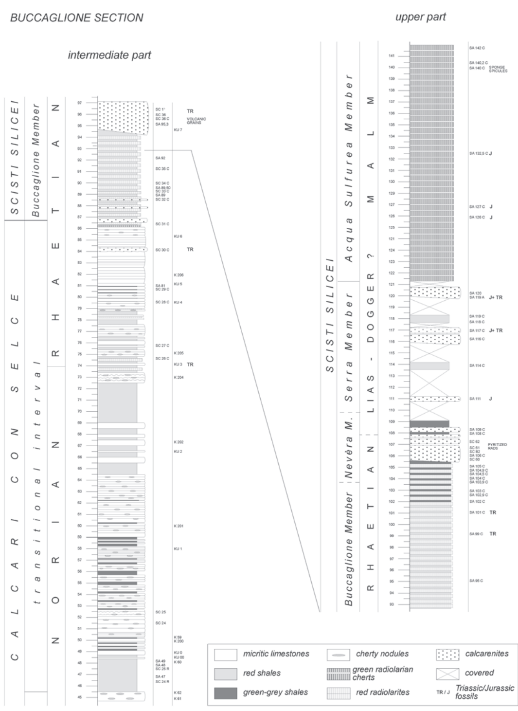
Passaggio dai Calcarei con Selce agli Scisti Silicei nella sezione del M. Buccaglione.
