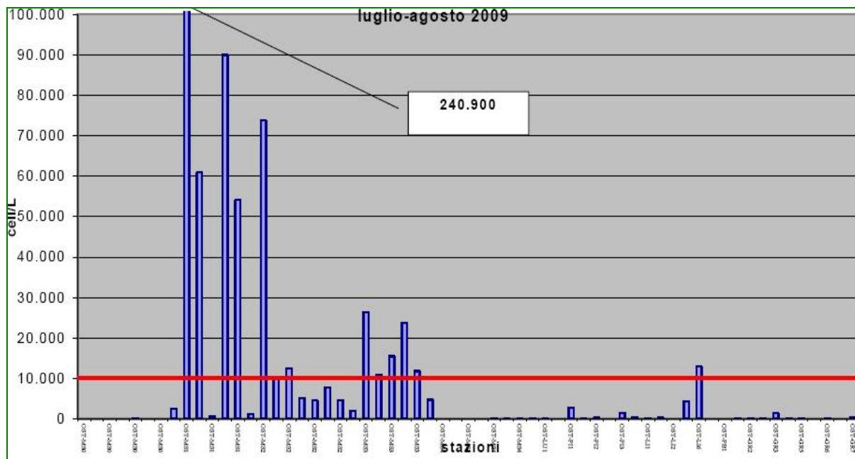
Figura 14.34 – Andamento di O.ovata in colonna d'acqua nei mesi di luglio e agosto lungo il litorale toscano – Anno 2009
