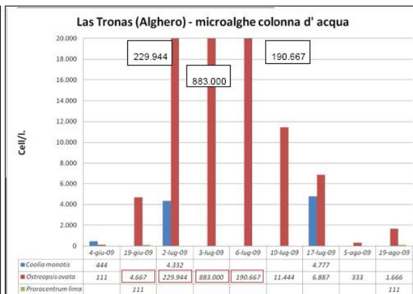
Figure 12.4 e 12.5 – Concentrazine delle microalghe su substrato e in colonna d’acqua (Dati MATTM)
