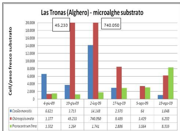
Figure 12.4 e 12.5 – Concentrazine delle microalghe su substrato e in colonna d’acqua (Dati MATTM)
