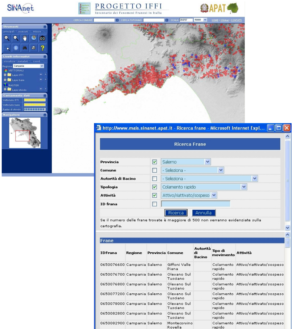
Figura 4.5 Funzione Query.
