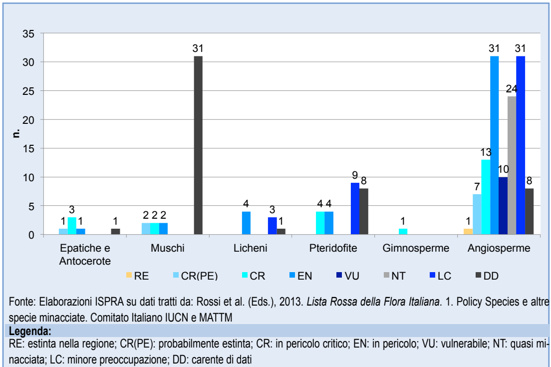
Figura 8.12: Numero di policy species presenti in Italia per ciascun gruppo sistematico e per categoria di rischio
