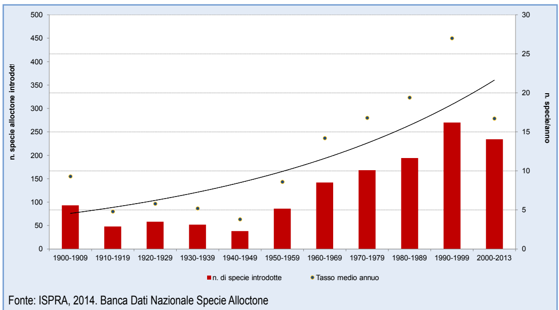
Figura 8.17: Numero di specie introdotte in Italia a partire dal 1900 e tasso medio annuo di nuove introduzioni, calcolati su 1.383 specie di data introduttiva certa
