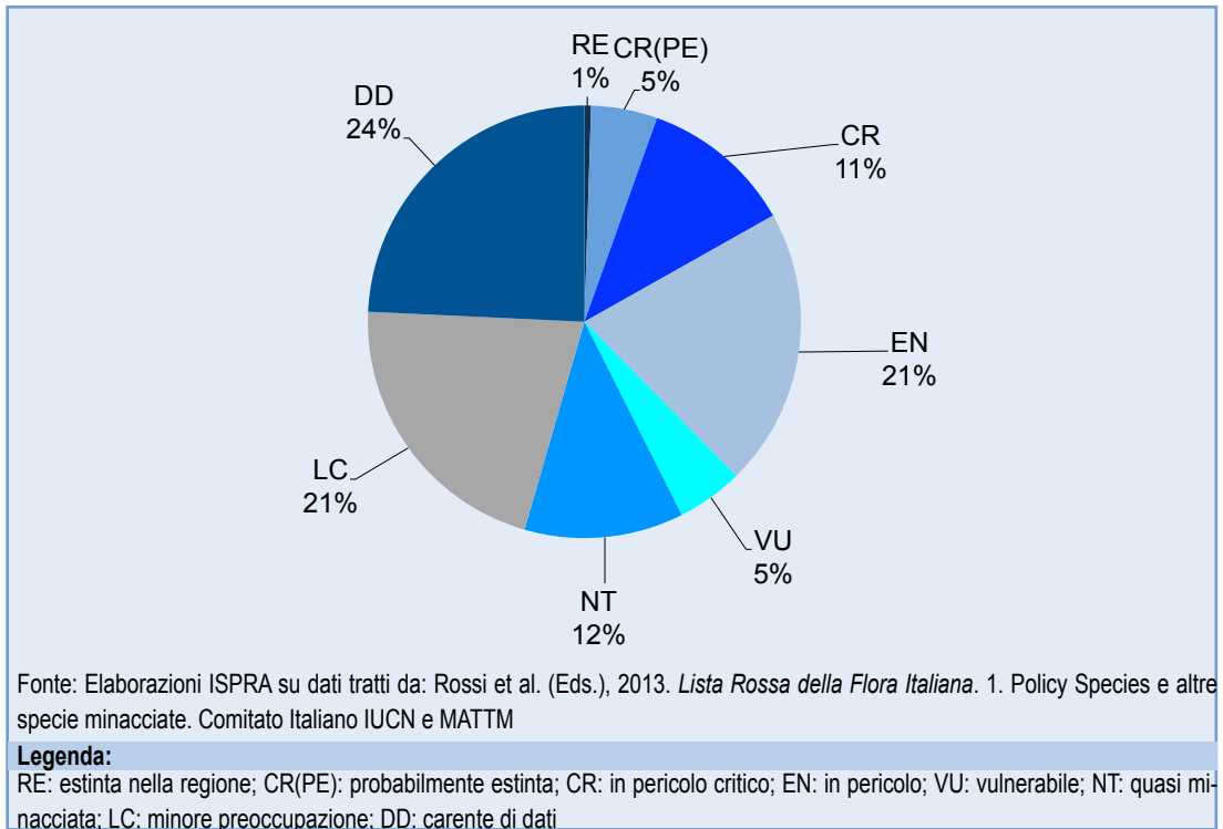
Figura 8.13: Ripartizione percentuale nelle categorie di minaccia IUCN (vers. 3.1) delle policy species
