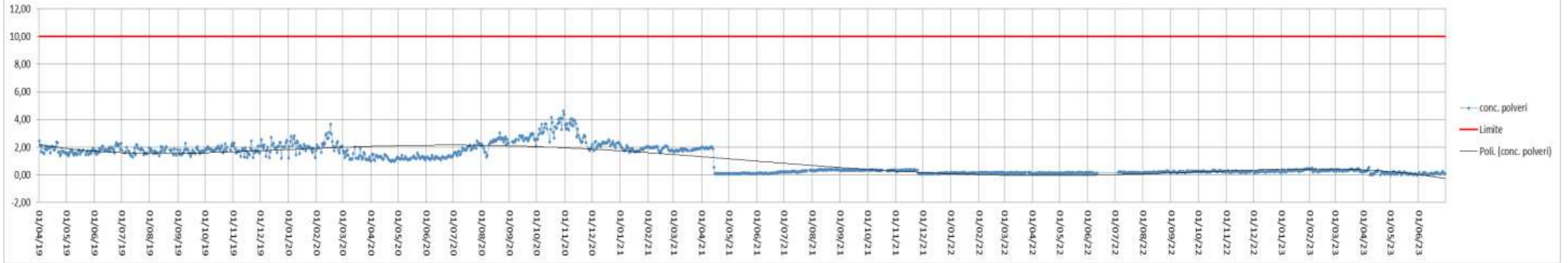
Polveri (mg/Nm3) camino E111
