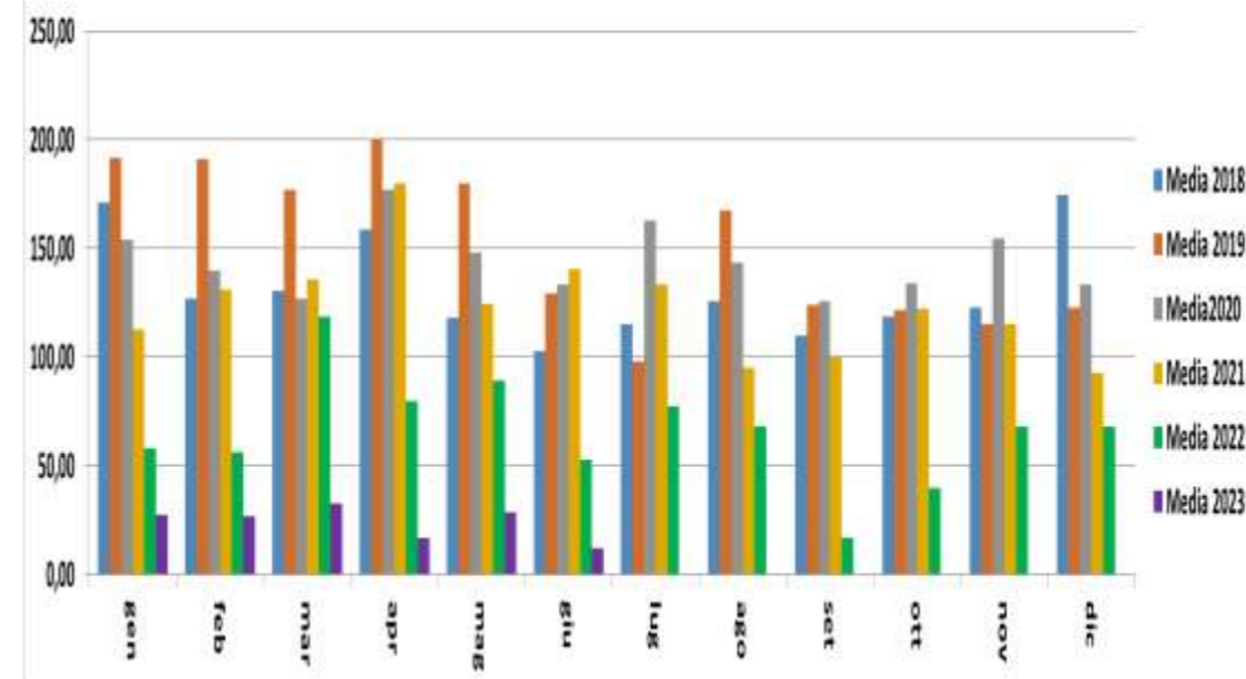
Concentrazione SOx (mg/Nm3) camino E312 medie mensili ANNI 2019-2020-2021-2022-2023 (I semestre)
