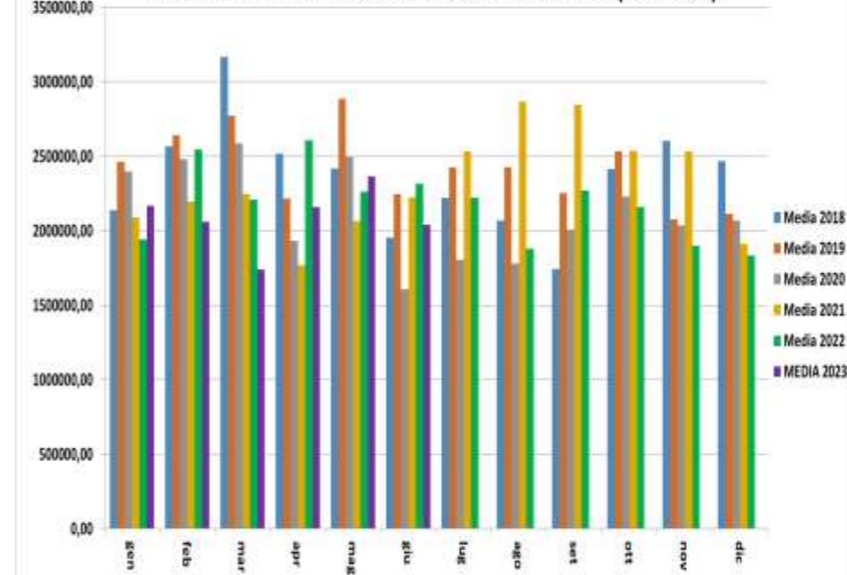
Portata fumi (Nm3/h) camino E312 medie mensili ANNI 2018-2019-2020-2021-2022-2023 (I semestre)
