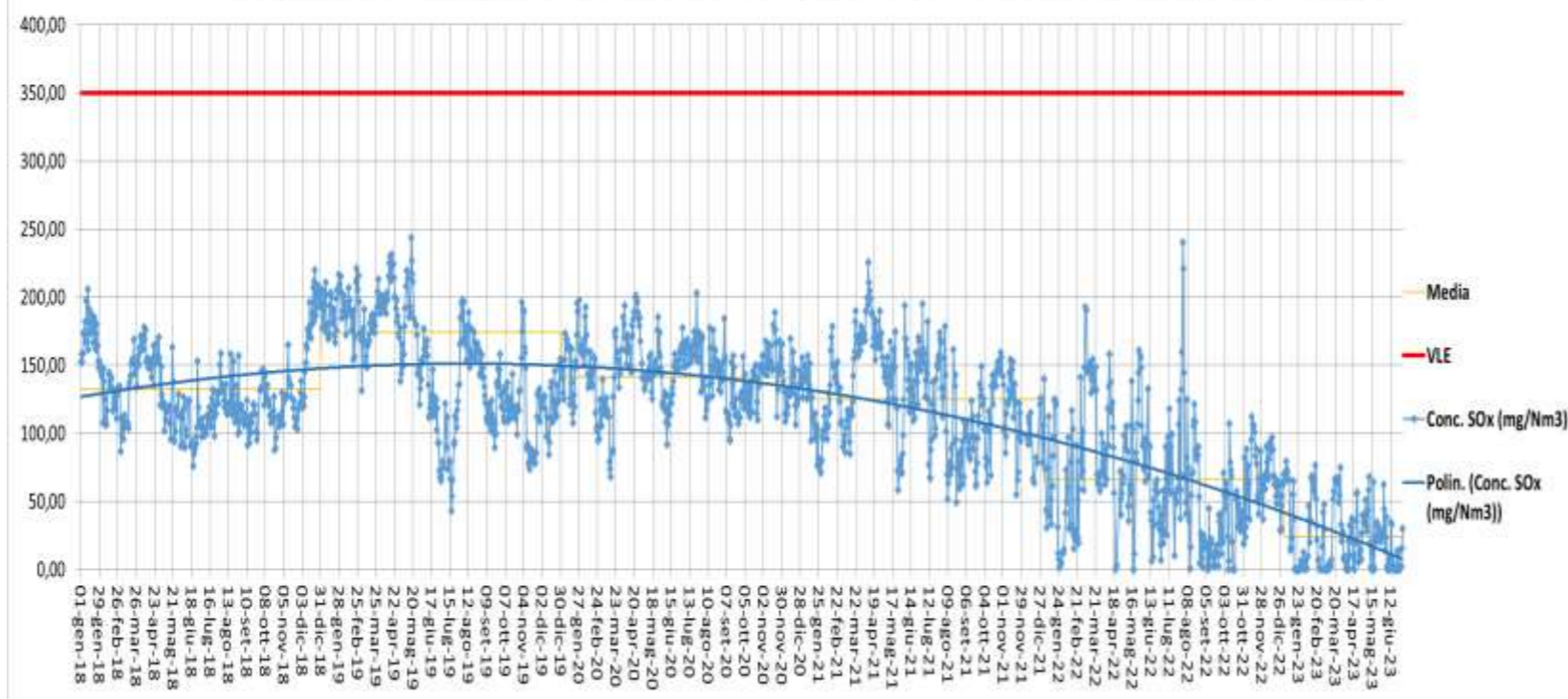
Concentrazione SOx (mg/Nm3) - Camino E312 - Anni 2018 - 2019 - 2020 - 2021 - 2022 - 2023 (I semestre)
