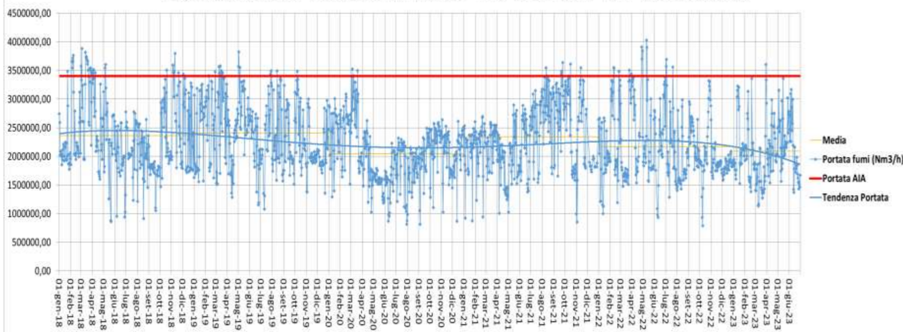
Portata fumi (Nm3/h) - Camino E312 - Anni 2018 - 2019 - 2020 - 2021 - 2022 - 2023 (I semestre)
