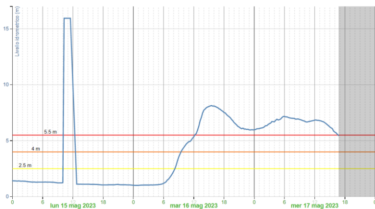
Figura 8 - Idrogramma di piena registrato alla stazione idrometrica di San Carlo sul Savio. FONTE ARPAE Emilia Romagna
