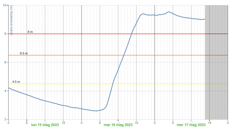
Figura 6 - Idrogramma di piena registrato alla stazione idrometrica di Ponte Braldo sul Montone. FONTE ARPAE Emilia Romagna
