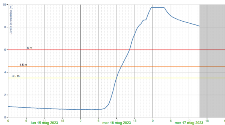
Figura 7 - Idrogramma di piena registrato alla stazione idrometrica di Faenza sul Lamone. FONTE ARPAE Emilia Romagna
