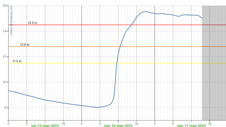
Figura 5 - Idrogramma di piena registrato alla stazione idrometrica di Sesto Imolese sul Sillaro. FONTE ARPAE Emilia Romagna
