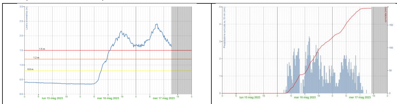
Figura 4 - Idrogramma di piena registrato alla stazione idrometrica di S. Ruffillo Savena e pluviogramma alla stazione di Monghidoro parte alta del bacino del Savena. FONTE ARPAE Emilia Romagna
