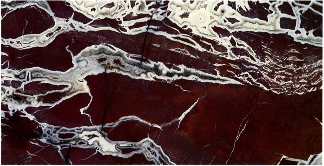
FIG. 33. - Campione 33 : DIASPRO ROSSO RADICELLATO AGATATO - Diaspro
