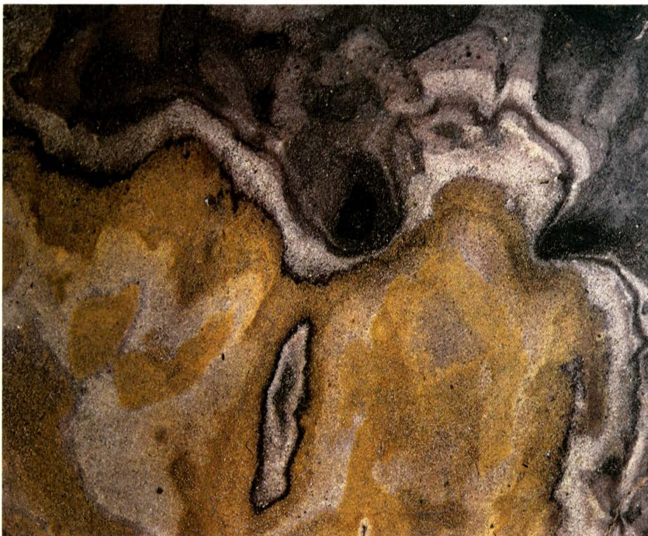
FIG. 58. - Campione 58: DIASPRO « DI SIBILIO » ZOOMORFO VARICOLORE ZONATO ( Lapis zoomorphus ) - Arenaria
