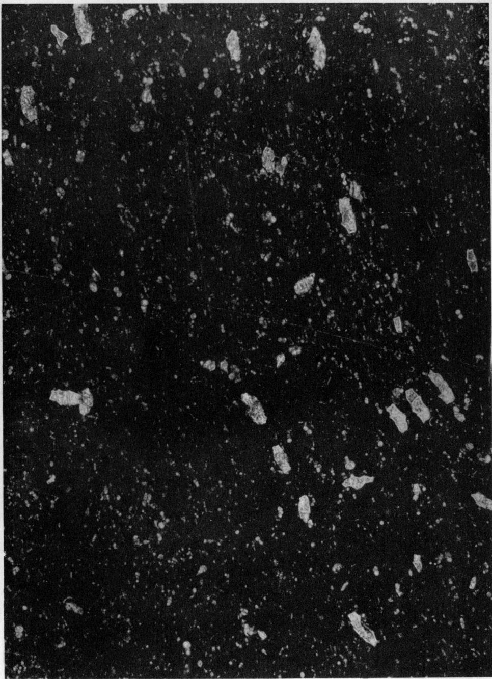
Fig. 2. Scaglia con Globotruncana linnei (D'ORB.) = Zona 1 a''.
