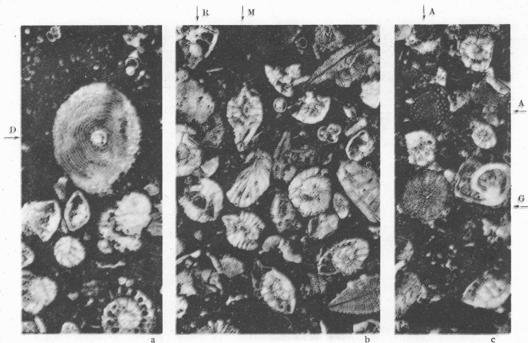
1 a : Discocyclusina cf. seunesi (H. Douv.) (D) e rotaliidi. Prof. XIX, Strato 16 ; b : Miscellanea cf. miscella (D' ARCH.) (M) e rotaliidi (R). Prof. XIX, Strato 21 ; c : Gypsina globulus REUSS (G) e Alveolina sp. (A). Prof. XIX, Strato 12. Tutte : 14 x.
