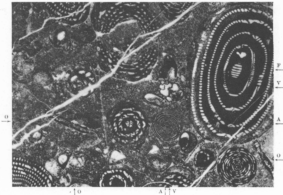
2. Ciottoli di calcare ad alveoline (Ypresiano) del M. Torretta (Prof. XXI/2 Strato 3) con Alveolina sp., A. minutula REICHEL (A) (pag. 161), Alveolina ( Flosculina sp.) (F), Orbitolites complanatus LAM. (O), valvuline (V). 14 x.
