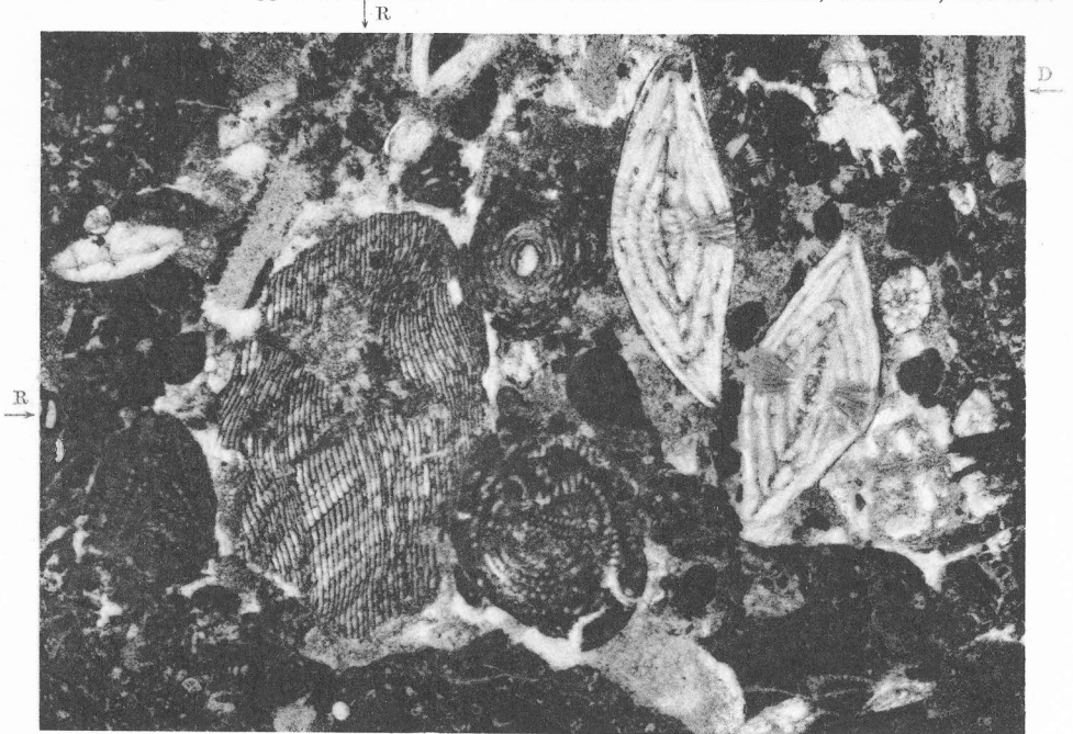
1. Eocene medio della loc. Il Poggiolo, con nummuliti radiate, alveoline consumate, discocycline (D) e frammenti di rudiste fluitate (R). 14 ×.
