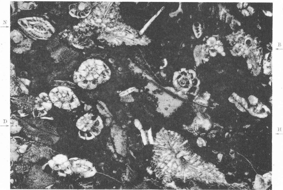
2. Calcare a baculogypsine dell' Eoc. sup. ( B. meneghinii var. tetraedra SILV. (B) con discocycline (D), piccole nummuliti radiate (N), rotaliidi e Halkyardia (H). Prof. XXIV, Strato 12. 14 ×.
