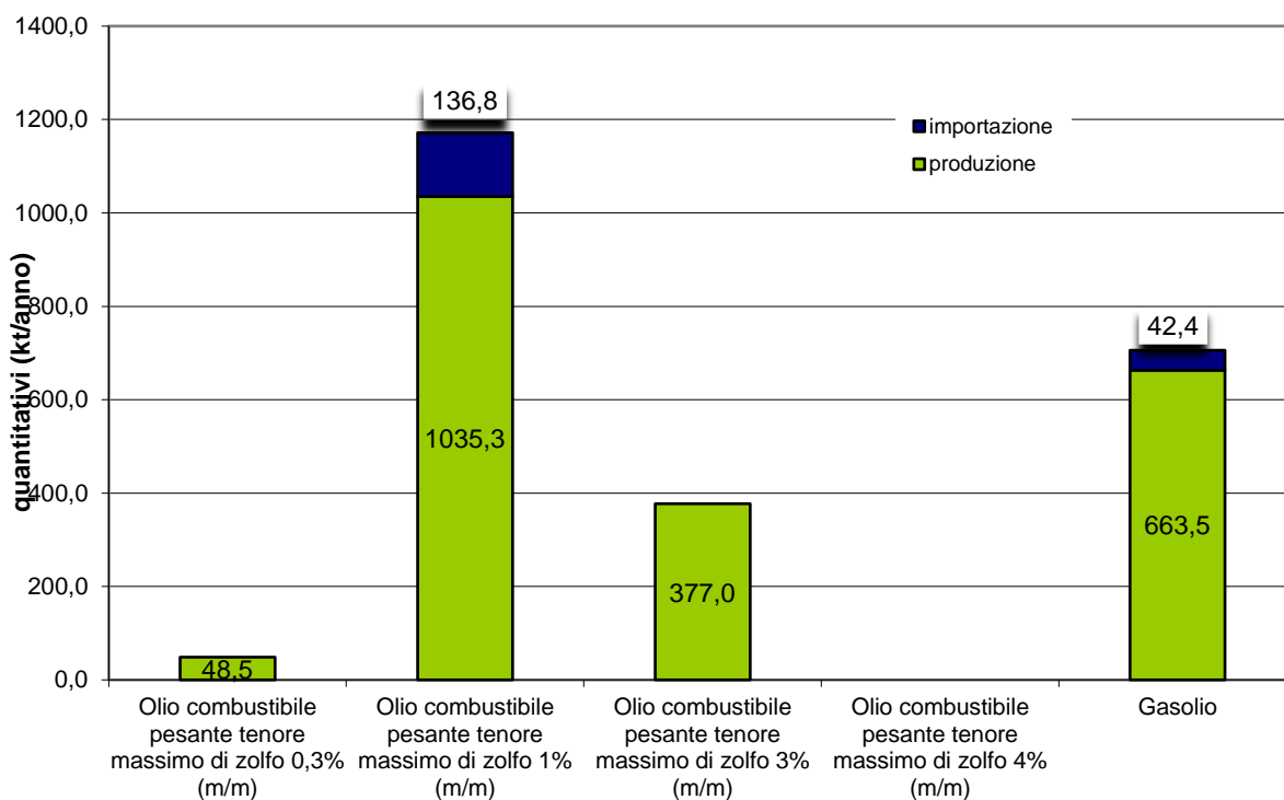
Fig. 4.1 Quantitativi di olio combustibile pesante e gasolio prodotto e importato nel 2021 con l'esclusione dei quantitativi destinati all'esportazione e l'inclusione dei quantitativi utilizzati nell'interno dell'impianto
