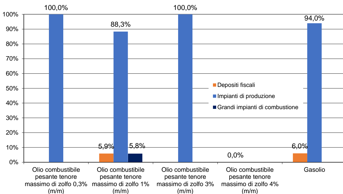
Fig. 4.4 Olio combustibile pesante e gasolio prodotti e importati nel 2021, con l'esclusione dei quantitativi destinati all'esportazione e l'inclusione dei quantitativi utilizzati all'interno dell'impianto. Ripartizione percentuale in funzione del tipo di olio e del tipo di impianto
